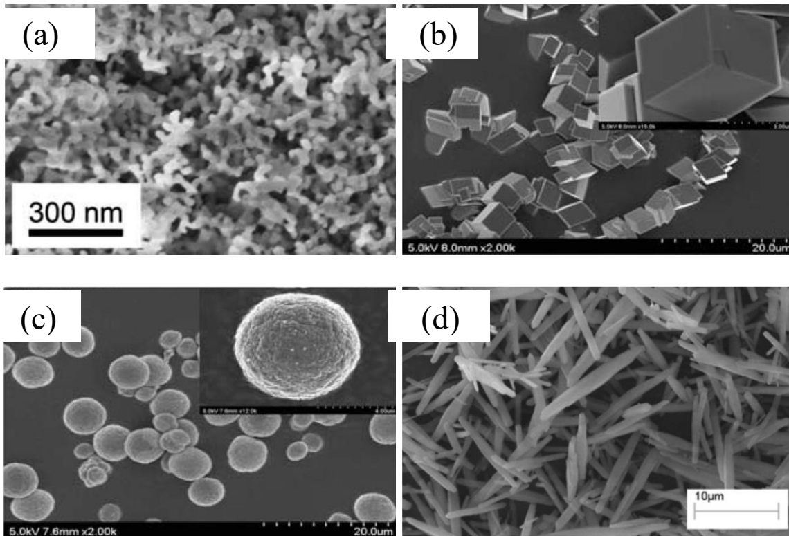
Fig. 1. Polymorphs of CaCO 3 . (a) Amorphous calcium carbonate (ACC) (Rodriguez-Blanco et al., 2011); (b) calcite (Chu et al., 2013); (c) vaterite (Chu et al., 2013); (d) aragonite (Zhou et al., 2004)
