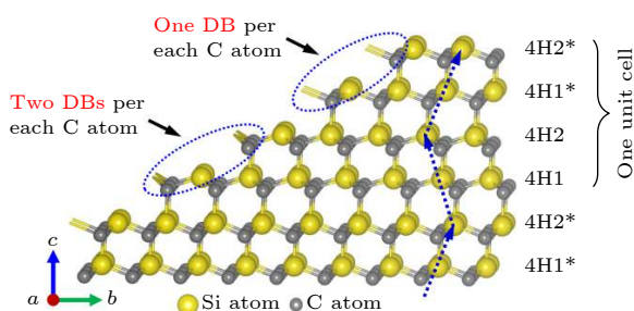
图 15 4H-SiC(0001) 表面台阶结构的键结构 (观察方向 [1120]) [64]
