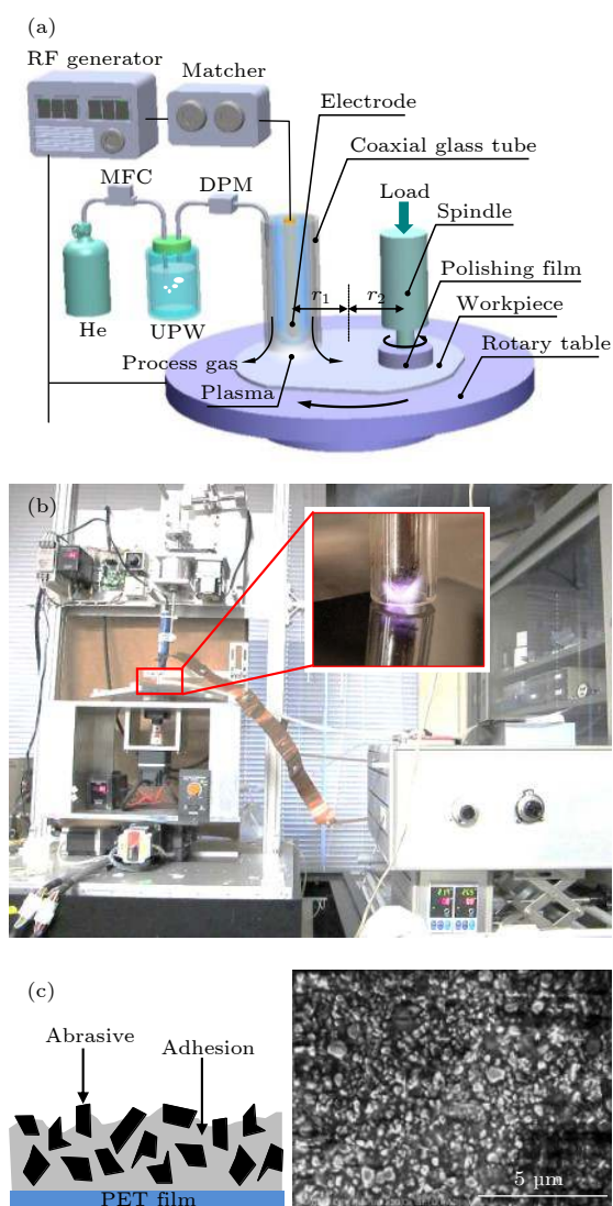
图 2 PAP 加工装置 (a) 装置示意图 [40] ; (b) 装置实物图 [45] ; (c) 抛光垫截面图及 SEM 图 [45]
