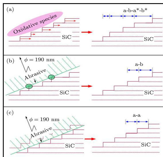
图 16 4H-SiC 台阶状结构形成机制 [65] (a) 化学改性占主导机制, 产生 a-b-a*-b*型结构; (b) 化学改性作用与磨粒物理去除作用相当, 产生 a-b 型结构; (c) 磨粒物理去除作用占主导机制, 形成 a-a 型结构
