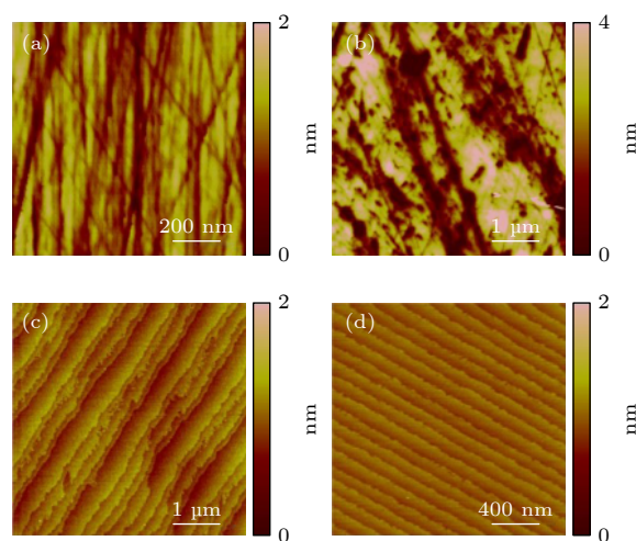
图 7 CMP 加工 SiC 的 AFM 图 (PV 表示最高和最低处的差值; RMS 是均方根) [45]: (a) 金刚石抛光液 (PV, 2.46 nm; RMS, 0.30 nm); (b) \text{Al}_2\text{O}_3 抛光液 (PV, 30.63 nm; RMS, 1.28 nm); (c) \text{SiO}_2 抛光液 (PV, 2.01 nm; RMS, 0.15 nm); (d) \text{CeO}_2 抛光液 (PV, 0.68 nm; RMS, 0.08 nm)
