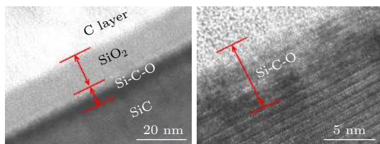
图 14 等离子体辐照后 4H-SiC 样品表面的 XTEM 图 [45]
